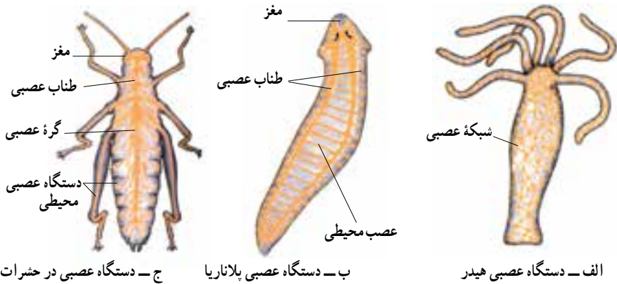
شکل ۱۶-۲- دستگاه عصبی چند جانور
