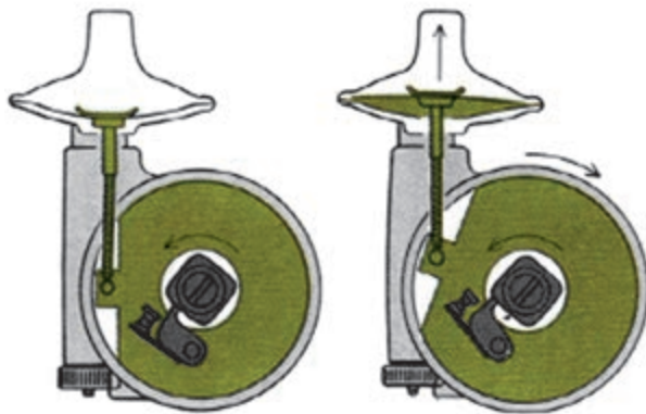
شکل ۲۹- ۱۰- نحوه‌ی عمل دستگاه آوانس خلی
