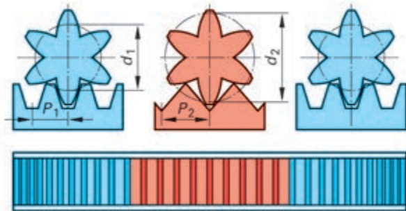
شکل ۱۰-۲- انواع پنیون و دنده شانه‌ای
