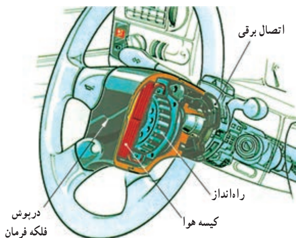
شکل ۲۱-۲- فلکه فرمان با کیسه هوا (Air bag)
