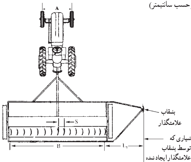
شکل ۱۸-۶- تنظیم علامتگذار
