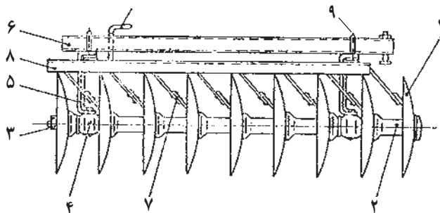
شکل ۵-۲- یک گروه بشقاب و نحوه اتصال آن به شاسی
