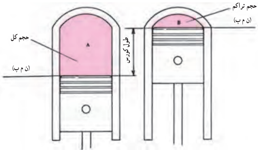
پیستون در نقطه مرگ بالا پیستون در نقطه مرگ پایین
