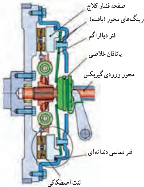
شکل ۱-۳- گروه انتقال قدرت (قسمت کلاچ)
