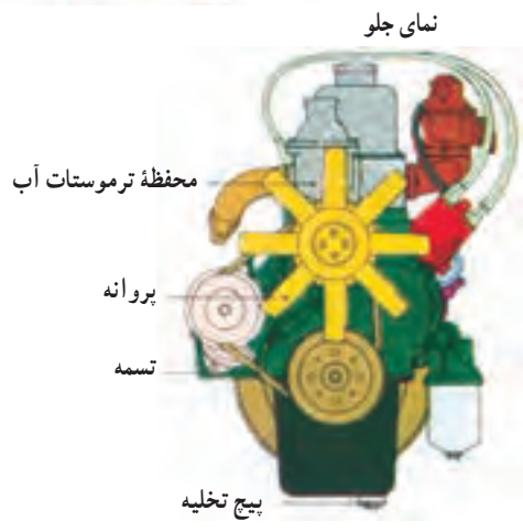
شکل ۱۱-۱ موتور در نماهای مختلف
