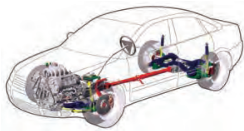
شکل ۱-۲- سیستم انتقال قدرت در یک خودرو
