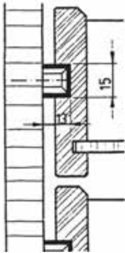
شکل ۲-۱۰۲ هدایت آویخته به بدنه (۳) ریل هادی پیچ شده به بدنه با وسیله حفاظت از بیرون افتادن جعبه
