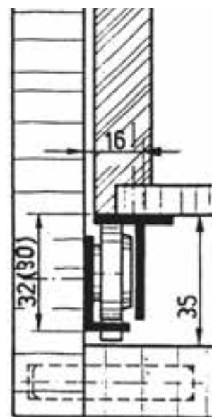
شکل ۲-۱۰۷- هدایت مکانیکی ساده (۴) با بلبرینگ
