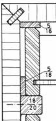
شکل ۲-۹۸- هدایت استاندارد (۵) به منظور استفاده بهتر از ارتفاع بدنه جعبه، آن را در قسمت بالا دو راهه زده‌اند که وظیفه قید جلوگیری از افتادگی و قید هادی بغل جعبه را انجام می‌دهد.
