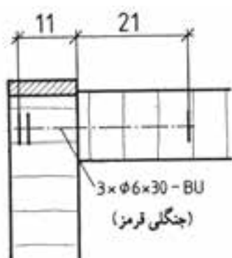
شکل ۲-۶۰- طریقه ترسیم دوپل ساده با خط محور
