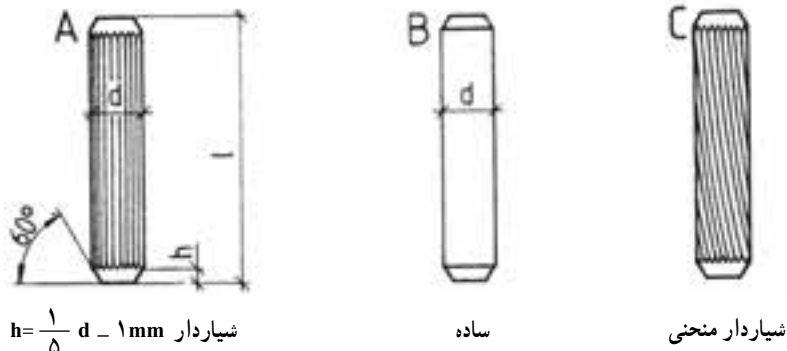
شکل ۲-۵۸- انواع دوپل‌ها
