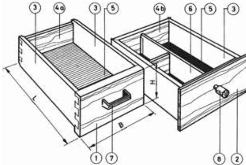
شکل ۸۷-۲- تصویر مجسم جعبه‌های استاندارد (کلاسیک) و قطعات مختلف آنها
