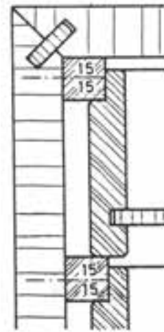
شکل ۲-۹۴- هدایت استاندارد (۳) قید هادی زیر بدنه جعبه بالایی همزمان به جای قید جلوگیری از افتادگی برای جعبه پایینی عمل می‌کند = قید هادی بغل جعبه و قید جلوگیری از افتادگی جعبه بالایی
