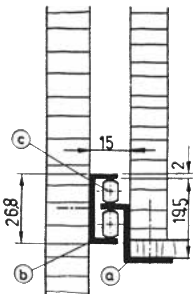
شکل ۲-۱۰۸- هدایت مکانیکی ساده (۳) با غلتک
