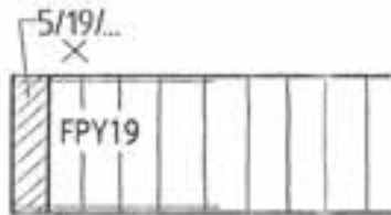
شکل ۲-۱۳ - علائم اختصاری تخته خرده چوب دو طرف روکش شده سرچوب با ضخامت ۱۹ میلی‌متر و زهوار ۵×۱۹ میلی‌متر
