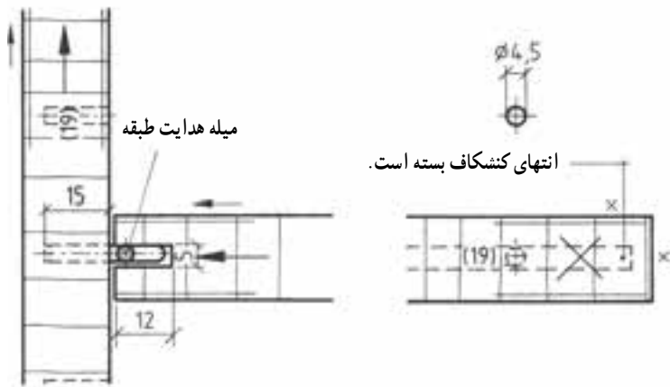
شکل ۲-۴۸. رسم پراق اتصال طبقه کابینت به وسیله زیر سری مفتول زبانه خم در تصویر مجسم و برش پیشانی و برش عمودی و کنشکاف از مفتول در انتهای عرض طبقه بسته است.
