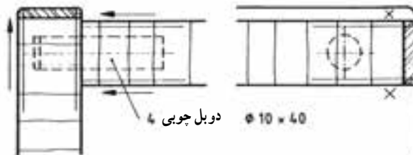
شکل ۲-۶۲- طريقة ترسیم اتصال دوبل در صفحات چوبی به وسیله ۴ دوبل به قطر ۱۰ mm و طول ۴۰ mm در برش نمای روبه‌رو و نمای پهلو با فاصله خالی
