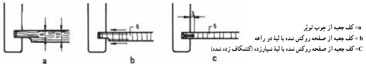
شکل ۲-۹۲- a تا c روش ترسیم اتصال کف جعبه به بدنه جعبه
