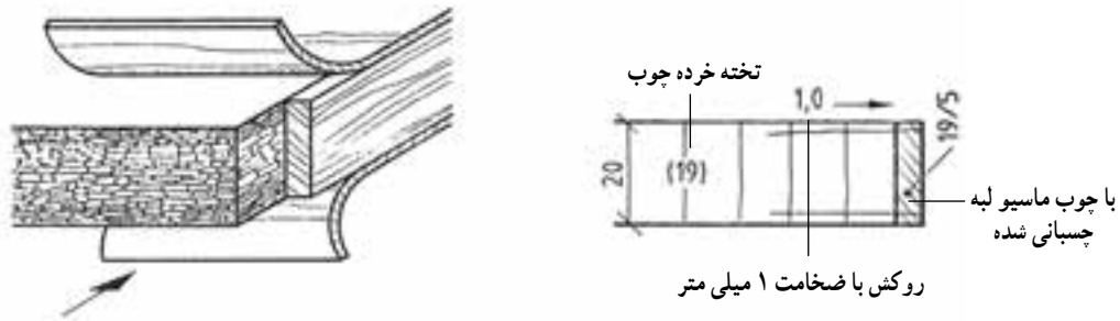
شکل ۲-۱۴ - تصویر مجسم و نقشه صفحه تخته خرده چوب به ضخامت ۱۹ میلی‌متر و زهوار لب چسبان به مقطع ۵×۱۹ میلی‌متر و دو طرف روکش کاج به ضخامت یک میلی‌متر
