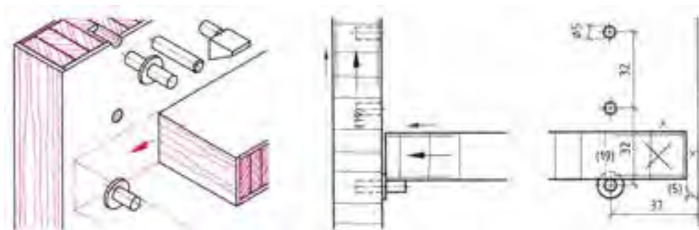
شکل ۸۱-۲ روش ترسیم نقشه اتصال طبقه به بدنه کابینت به وسیله زیرسری‌های استوانه‌ای و دوزنقه‌ای زبانه‌دار قابل تنظیم در برش پیشانی و نما با اندازه‌گذاری
