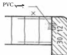
شکل ۲-۶۹- ترسیم علائم درز چسب با ۴ خط عمود بر امتداد درز
