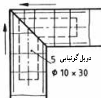
شکل ۲-۶۳- طريقة ترسیم دوبل گونیایی به قطر ۱۰ mm و به طول ۳۰ mm در برش
