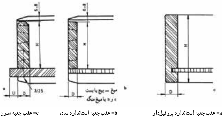
شکل ۹۱-۲- روش ترسیم انواع عقب جعبه‌ها
