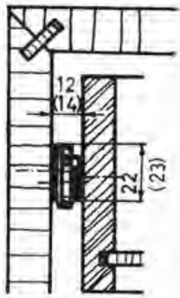
شکل ۲-۱۱۰- هدایت مکانیکی ساده (۱) با غلتک
