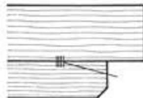
شکل ۶-۲- ترسیم هاشور راه چوب ماسیو قطعات به هم چسبیده
