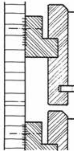
شکل ۲-۱۰۱ هدایت آویخته به بدنه (۲) قید هادی دو راهه شده این طرح وقتی به کار می‌رود که فاصله جعبه با بدنه زیاد باشد.
