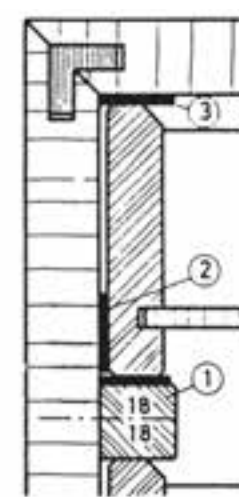
شکل ۲-۹۷- هدایت استاندارد (۶) ۱- قید هادی زیر بدنه بین جعبه‌ها یا قشر فشرده از مواد مصنوعی چسبانده شده ۲- قید هادی بغل جعبه ۳- قشر فشرده جهت جلوگیری از افتادگی جعبه
