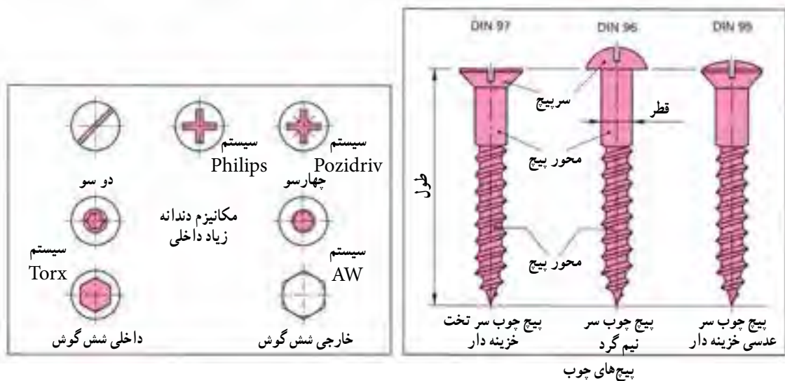
شکل ۲-۴۳- پیچ‌های چوب
