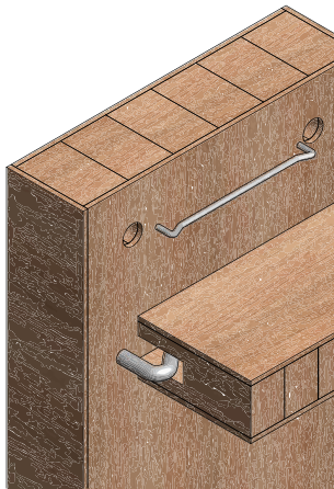
شکل ۲-۴۸. رسم پراق اتصال طبقه کابینت به وسیله زیر سری مفتول زبانه خم در تصویر مجسم و برش پیشانی و برش عمودی و کنشکاف از مفتول در انتهای عرض طبقه بسته است.
