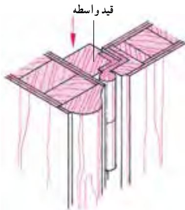
شکل ۲-۵۵- ترسیم لولای قابلمه‌ای سیلندری با در دو راهه شده و قید واسطه کابینت، زاویه باز شدن 10^\circ درجه
