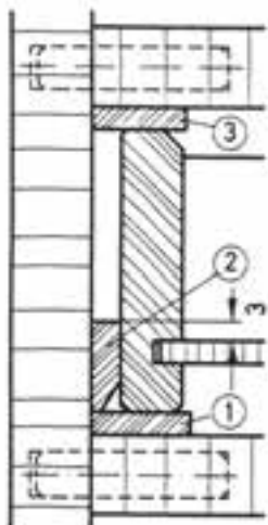
شکل ۲-۹۶- هدایت استاندارد (۱) ۱- قید هادی زیر بدنه ۲- قید هادی پهلوئی بدنه ۳- قید جلوگیری از افتادگی جعبه
