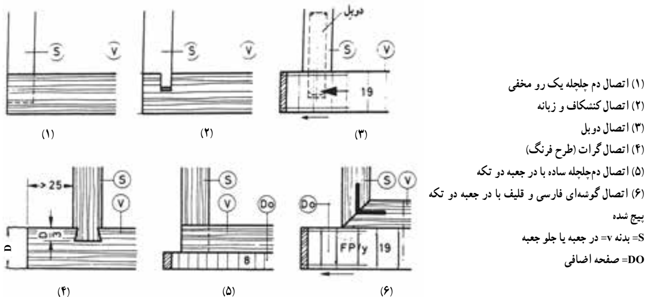
شکل ۸۹-۲- روش ترسیم انواع اتصالات در جعبه به بدنه جعبه در برش همراه با مشخصات مورد نیاز
