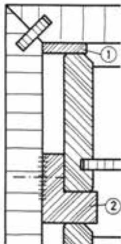
شکل ۲-۹۹- هدایت استاندارد (۴) ۱- قید جلوگیری از افتادگی ۲- قید دو راهه شده که برای جعبه بالایی وظیفه قید هادی بغل جعبه و قید هادی زیر بدنه و برای جعبه زیری قید جلوگیری از افتادگی را انجام می‌دهد.
