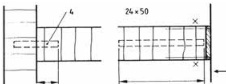
شکل ۲-۶۴- طريقة ترسیم اتصال قلیف زبانه کوتاه در صفحات چوبی به وسیله چهار زبانه کوتاه به عرض ۲۴ mm و طول ۵۰ mm در برش نمای روبه‌رو و نمای پهلو
