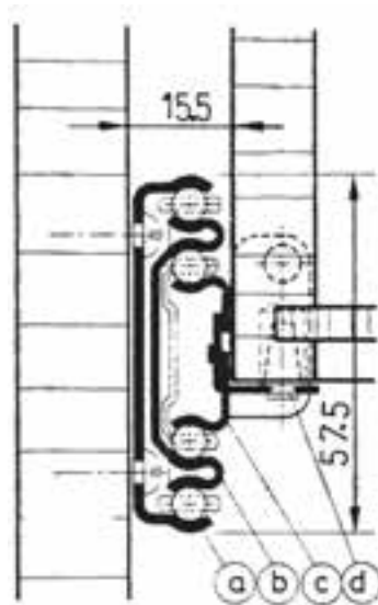
شکل ۲-۱۱۳- هدایت تلسکوپی
