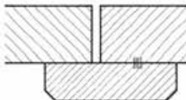
شکل ۷-۲- ترسیم هاشور سرچوب ماسیو قطعات به هم چسبیده
