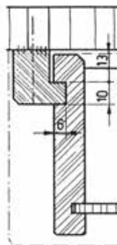
شکل ۲-۱۰۴ هدایت آویخته زیر سقف (۲) با قید هادی زبانه‌دار که در زیر سقف کابینت پیچ شده. هدایت جعبه در شکاف بدنه جعبه صورت می‌گیرد.
