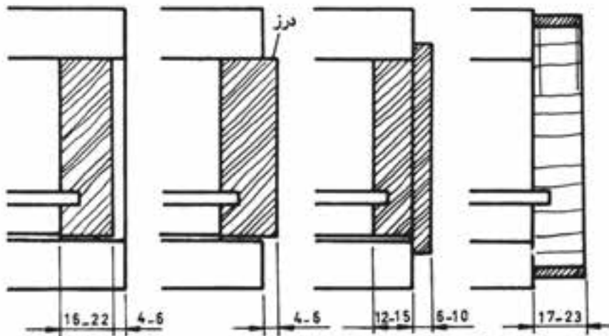
شکل ۸۸-۲- روش ترسیم حالت‌های قرارگیری در جعبه‌ها در برش، از چپ: در جعبهٔ تو نشسته، بیرون نشسته، رو نشسته دو تکه (یا دورا هه) و رو نشسته ساده
