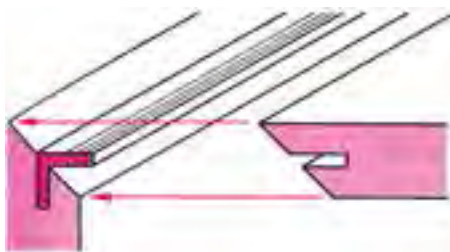
شکل ۲-۶۸- چگونگی استقرار زبانه مصنوعی در محل خود
