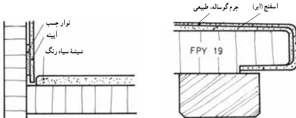
شکل ۲-۳۱- ترسیم علائم صفحات چوبی با نصب آینه و شیشه سیاه رنگ
