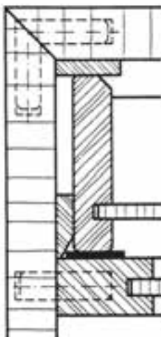
شکل ۲-۹۵- هدایت استاندارد (۲) به جای قید هادی زیر بدنه از قشر فشرده مواد مصنوعی استفاده شده است.
