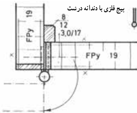
شکل ۲-۵۳ ترسیم لولای قدی زاویه باز شدن ۱۸۰ درجه
