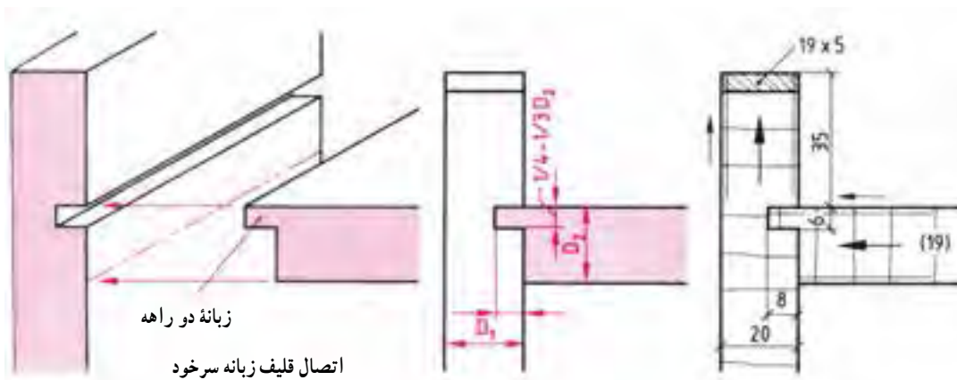
شکل ۲-۸۰- ترسیم علائم نقشه اتصال میانی صفحه به بدنه کابینت با قلیف زبانه سرخود به اندازه‌گذاری متناسب
