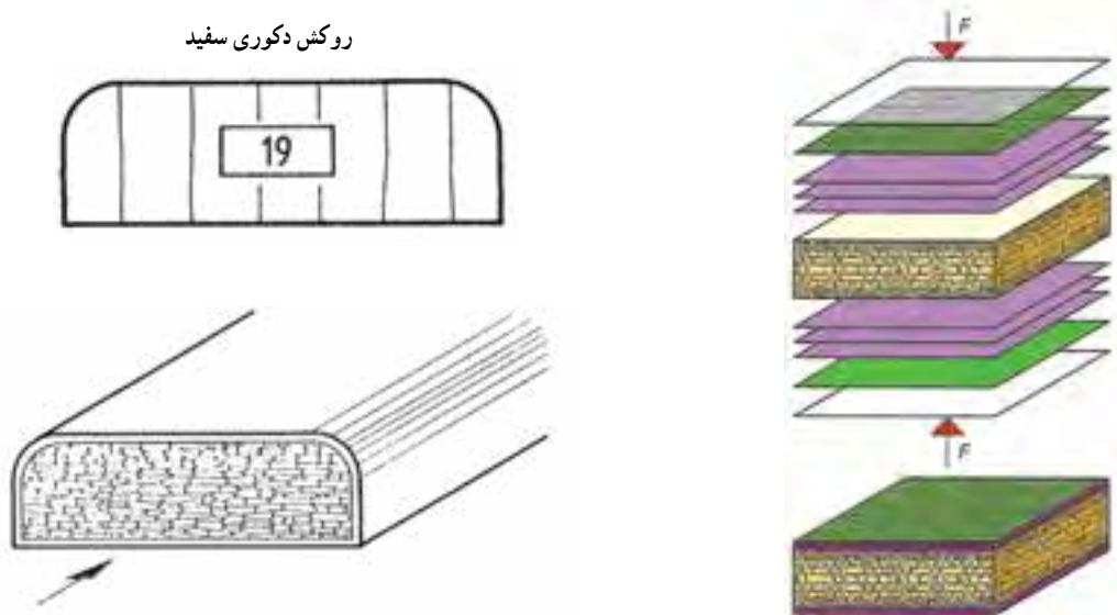
شکل ۲-۳۳- تصویر و نقشه صفحه تخته خرده چوب
