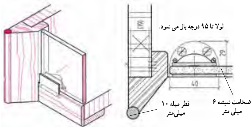
شکل ۲-۵۲ ترسیم نقشه در شیشه‌ای با لولای مخصوص که تا ۹۵ درجه باز می شود و قطر شیشه ۶ میلی متر است
