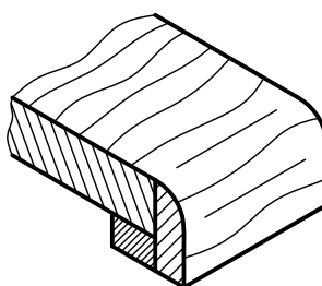
شکل ۳-۲- هاشور ۳ قطعه چوب ماسیو (توبر) کنار هم با نمایش سطح برش فرضی داده شده است
