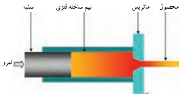
شکل ۸-۲۵- فرآیند اکستروژن در تولید قطعات صنعتی
