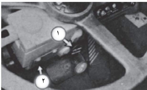
شکل ۲۷-۴ — تنظیم فرمان
