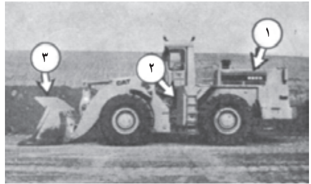
شکل ۳-۴- اجزای اصلی لودر
