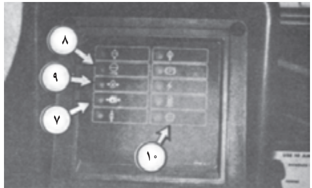
شکل ۱۱-۴ صفحه هشداردهنده
