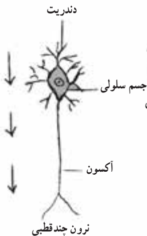
شکل ۲-۳- انواع نرون
