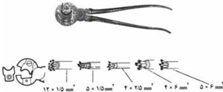
قیچی کابل بری و کابل‌های مربوط به آن
