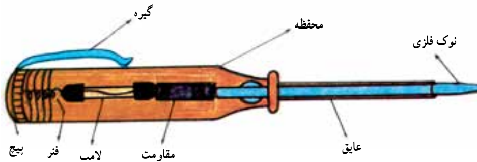
شکل ۲-۴- شمای ظاهری و ساختمان داخلی فازمتر
