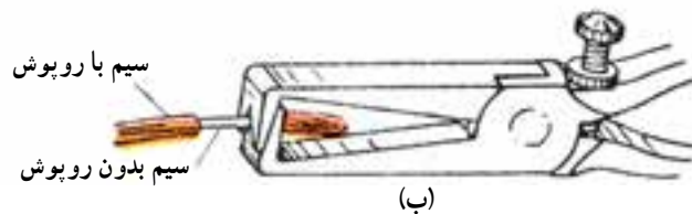
شکل ۱۱-۲- الف - تصویر ظاهری چند نوع سیم لخت کن ساده ب - تصویر یک سیم لخت کن ساده در حال لخت کردن سیم
