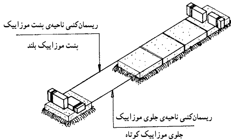
شکل ۱۸-۹- دلیل‌گذاری با اجرای شیب
