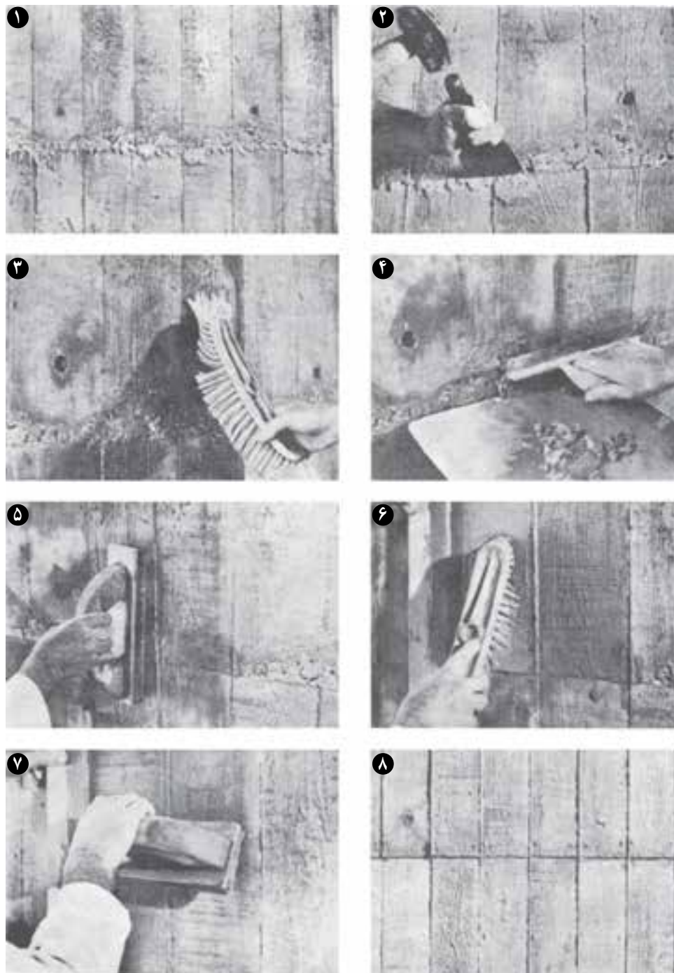
شکل ۶-۴۲- روش ترمیم دوغاب‌های اضافی که از محل درز بین دو قالب بیرون زده است.
