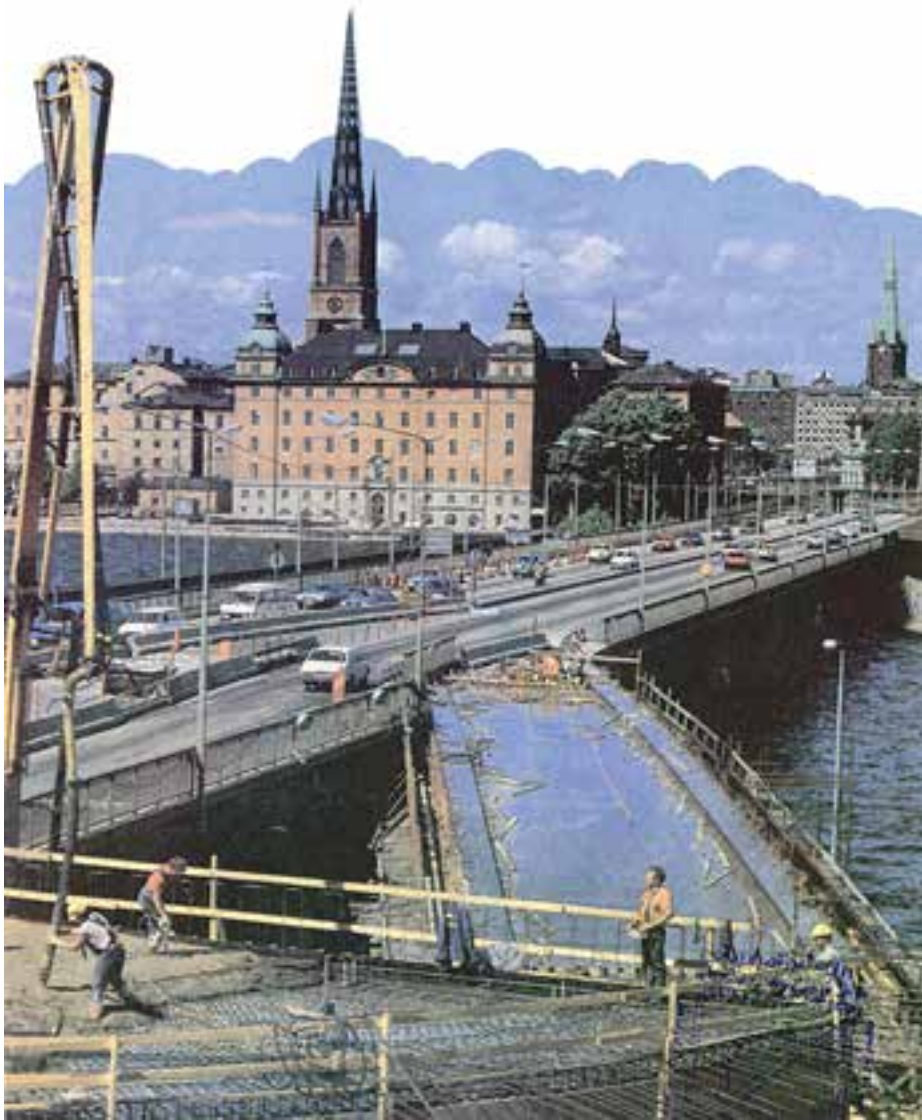
شکل ۶-۷- بتن آماده، در حال تخلیه به وسیله پمپ نصب شده بر روی کامیون
