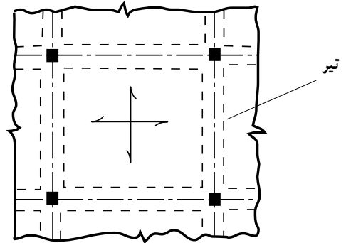
ب) دال دو طرفه
