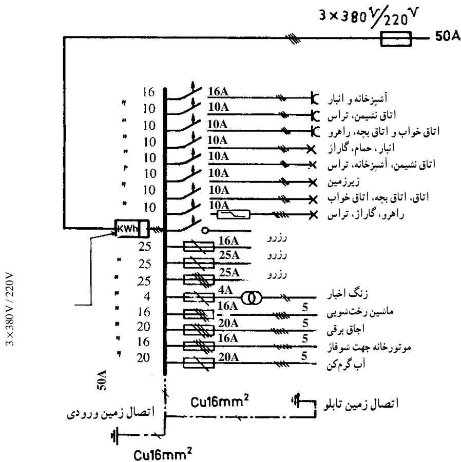
شکل ۲-۷ شمای فنی مدار الکتریکی یک تابلوی توزیع مربوط به ساختمان ویلایی در یک مزرعه
