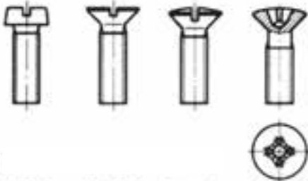
شکل ۴-۳ پیچ‌های شیاردار
