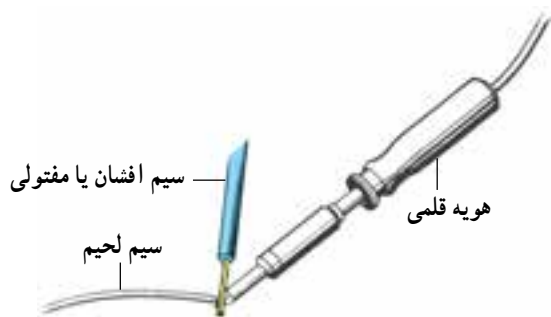
شکل ۴۰-۴ اصول صحیح قلع اندود کردن سرسیم
