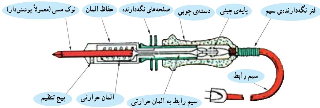
شکل ۳-۳۱ قسمت‌های مختلف یک هویه‌ی قلمی
