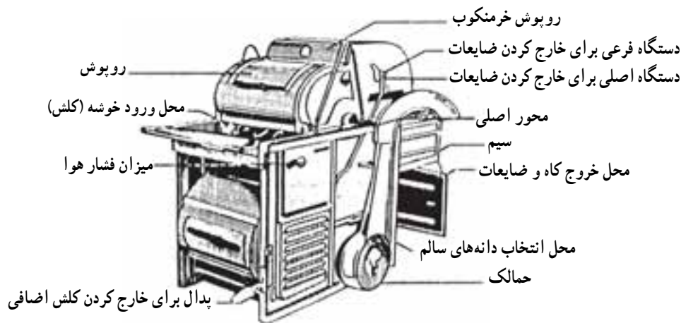
شکل ۲۲-۱- ساختمان خرمنکوب
