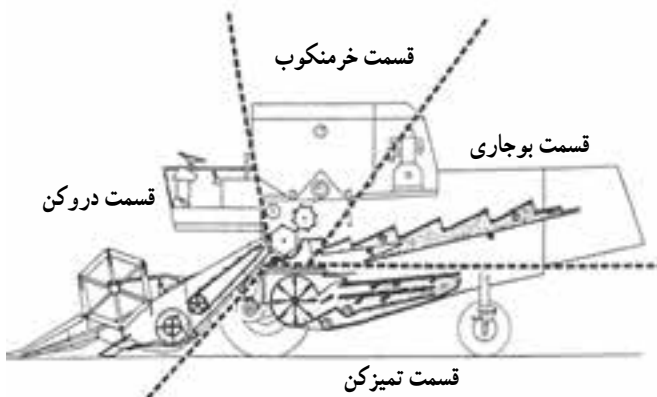
شکل ۱۹-۱- قسمت‌های داخلی کمباین
