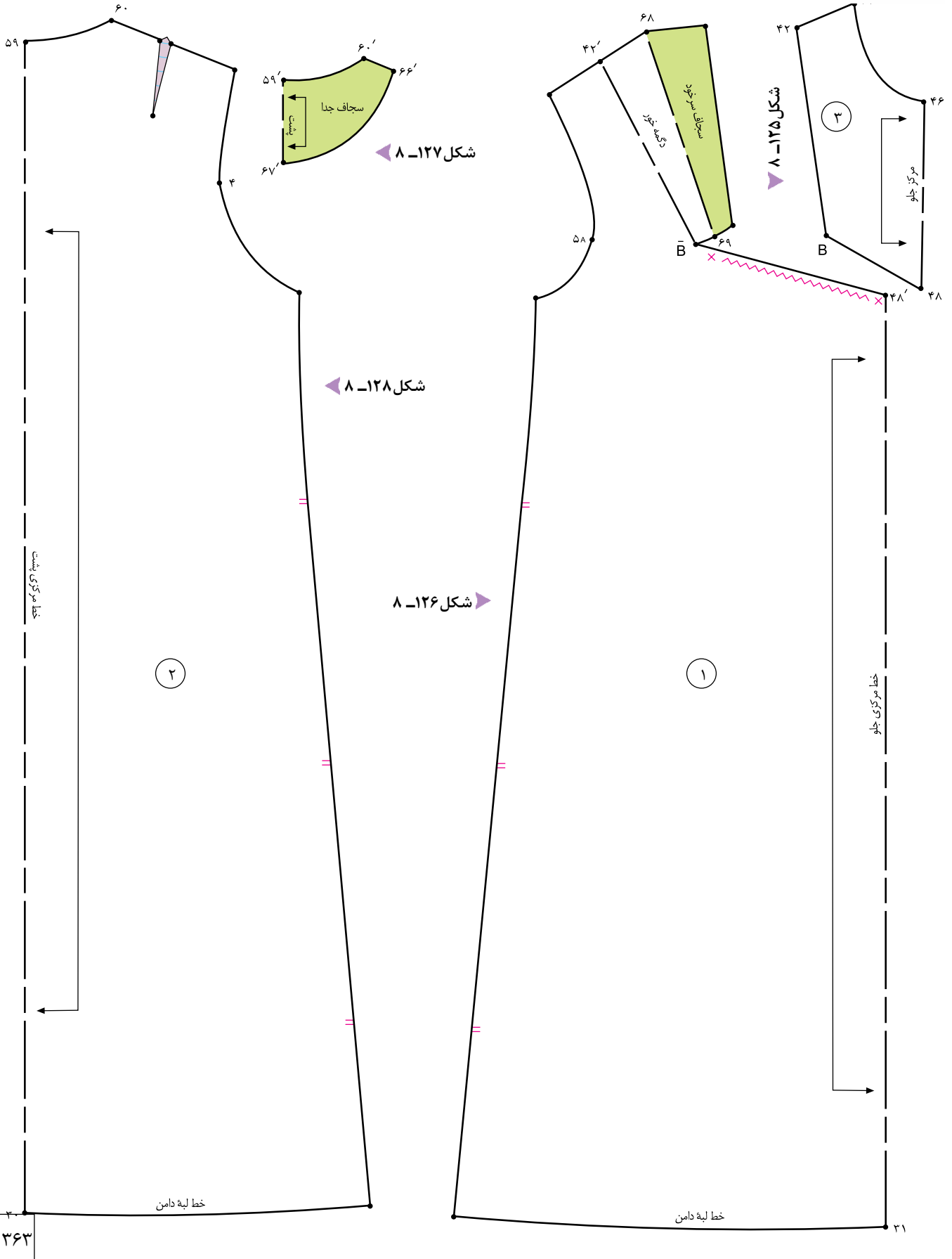
روی قطعات الگو علامت‌های راستای پارچه و موازنه را مشخص کنید. (شکل ۱۲۶، ۱۲۷، ۱۲۸ و ۱۲۵-۸)
