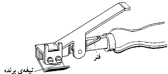
شکل ۲۴-۵- شیار درآر طولی کابل
