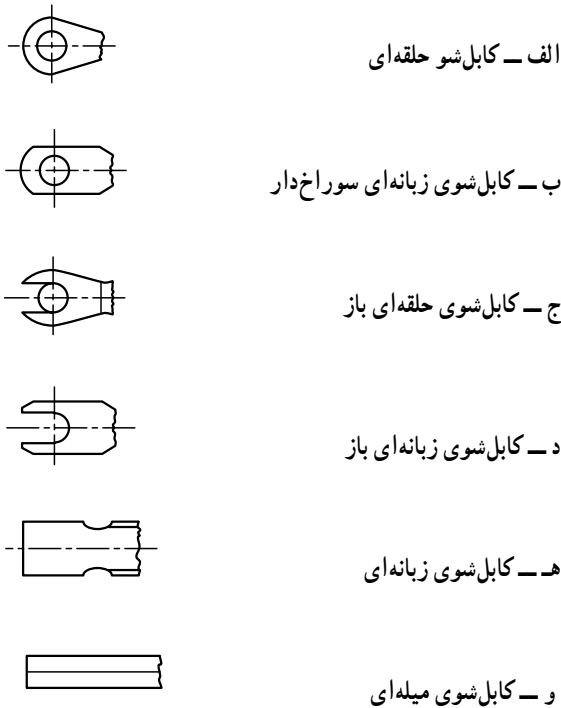
شکل ۲-۲۱- انواع کابل شوی پرسی
