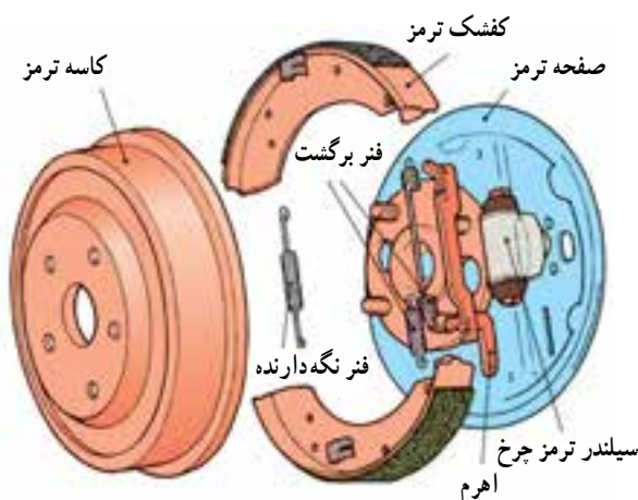
شکل ۳۵-۱- ترمز کفشکی
