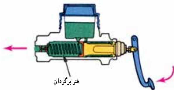
شکل ۱۹-۱- فنر برگردان پیستون
