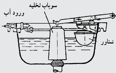
شکل ۱۲-۸- جزئیات سیفون مرتفع
