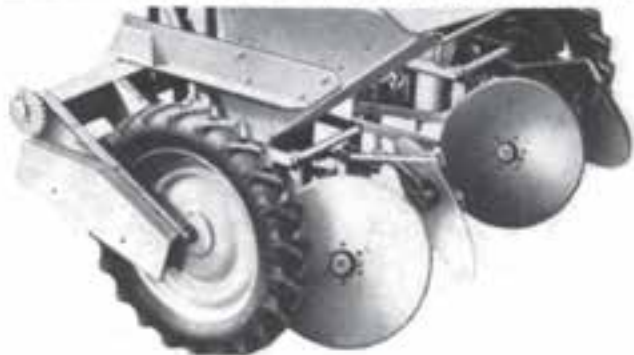
شکل ۶-۱۱ خاک دادن پای بوته‌ها
