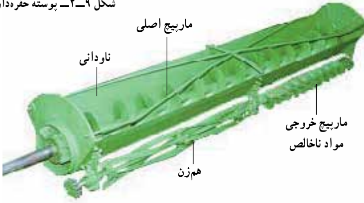
شکل ۲-۱۰ - اجزای داخلی استوانه حفره‌دار
