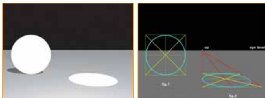
تصویر ۶-۱۲- شکل دایره هم در حالت تخت و هم در حالت عمق نمایی
