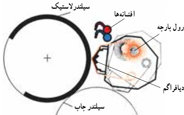
شکل ۳-۶- نمای سیستم شست و شوی اتوماتیک
