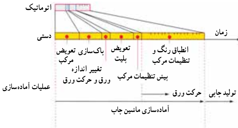
شکل ۱-۶- مقایسه‌ی زمان‌های آماده‌سازی دستی و اتوماتیک تولید یک کار چاپی چند رنگ
