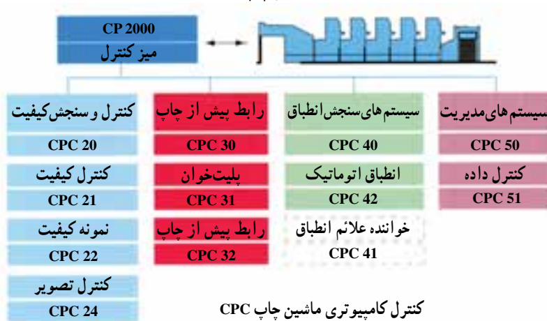
مرکز کنترل ماشین چاپ CP 2000
