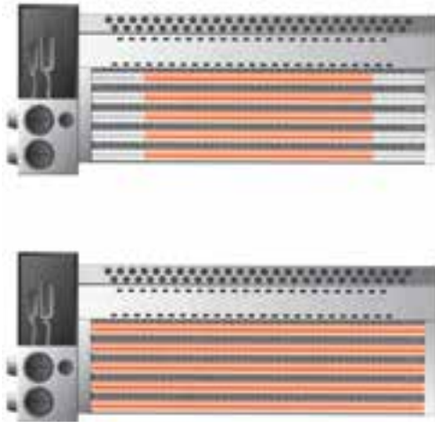
شکل ۳۹-۴- تطابق بهنای تابش اشعه نسبت به اندازه‌ی ورق چاپی
