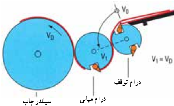
شکل ۴-۱۳- سیستم درام توقف
