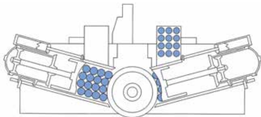
شکل ۱۲-۳- دستگاه خردکن
