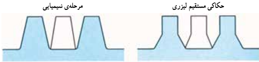
شکل ۳-۳- مقایسه‌ی ایجاد نقش برجسته‌ی یک پلیت چاپ فتوپلیمر تولید شده در یک مرحله‌ی فتوگرافیک / شیمیایی با پلیت (لاستیکی) حکاکی شده توسط لیزر
