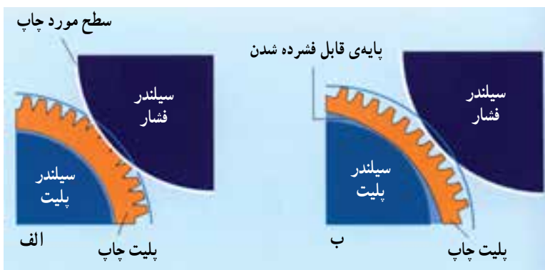
شکل ۳-۷- انتقال تصویری در فلکسوگرافی. الف) تغییر شکل پلیت چاپ، پلیت تک لایه، ب) انتقال مناسب تصویری با استفاده از یک پلیت چاپی با پایه‌ی فشارپذیر
