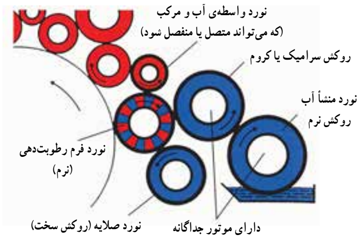
شکل ۱۱-۲- سیستم رطوبت‌دهی پیوسته
