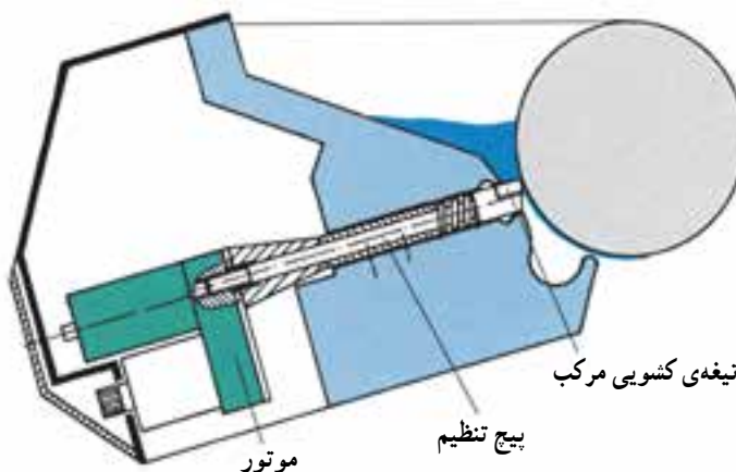
شکل ۱۵-۲- سیستم مرکبدان تیغه‌ی کشویی (RCI/CCI، مان رولند)
