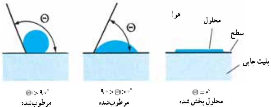
شکل ۱-۲- قابلیت رطوبت‌پذیری سطوح و زاویه‌ی رطوبت‌پذیری
