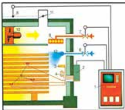
شکل ۱۳-۳- اجزای سیستم اتوماتیک کنترل کوره
