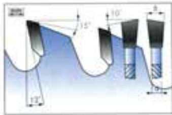
شکل ۱-۳۰ تیغه اره اونیورسال
