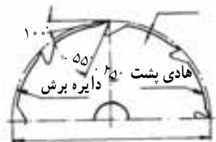
تیغه اره گرد به نام ویگو برای برشهای طولی و عرضی در چوبهای نرم
