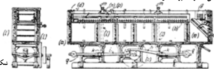
نمای شماتیک جیگ هان کاک
