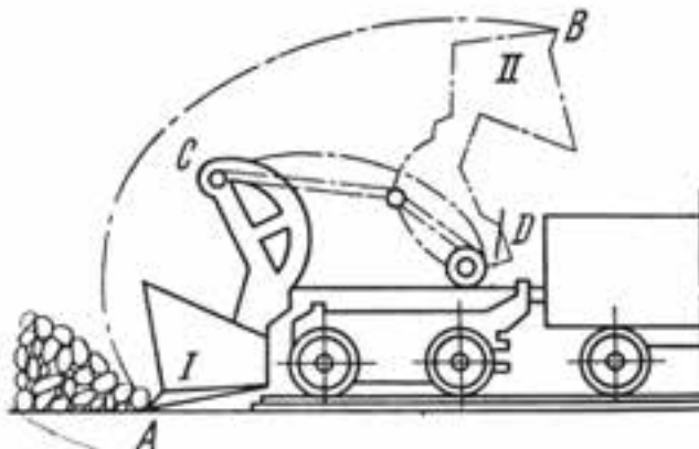
شکل ۱-۱۰- بارکننده مکانیکی [۲]
