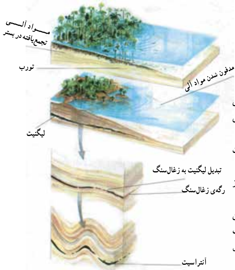
شکل ۱۴-۱۱- تشکیل زغال سنگ از رسوبات مردابی
