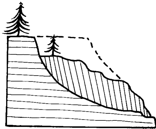
الف) زمین لغزه‌ای که در آن سطح لغزش منحنی است.
