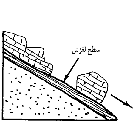
ب) وجود لایه‌ی رسی که سبب لغزش سنگ‌ها و قطعات بالایی می‌شود.
