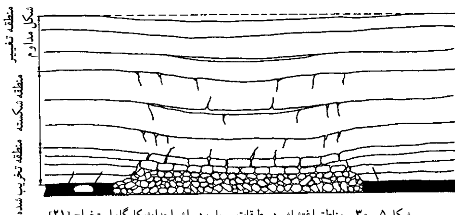
شکل ۵-۳- مناطق اغتشاش در طبقات روباره در اثر احداث کارگاه استخراج [۲۱]
