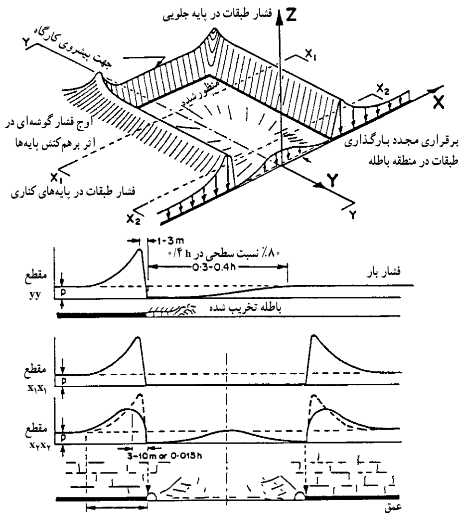
شکل ۵-۲۹- توزیع تنش در پایه‌های اطراف یک بهنه زغالی ایالات متحده آمریکا [۲۱]
