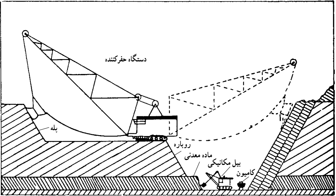
شکل ۳-۱- نمایی از یک معدن روباز [۱]
