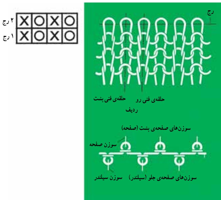
شکل ۱۰-۲۱- ساختمان بافت ریب ۱.
