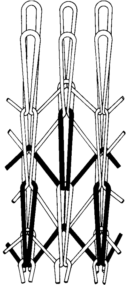
شکل ۱۰-۳۲- ساختمان بافت پیکه تکی
