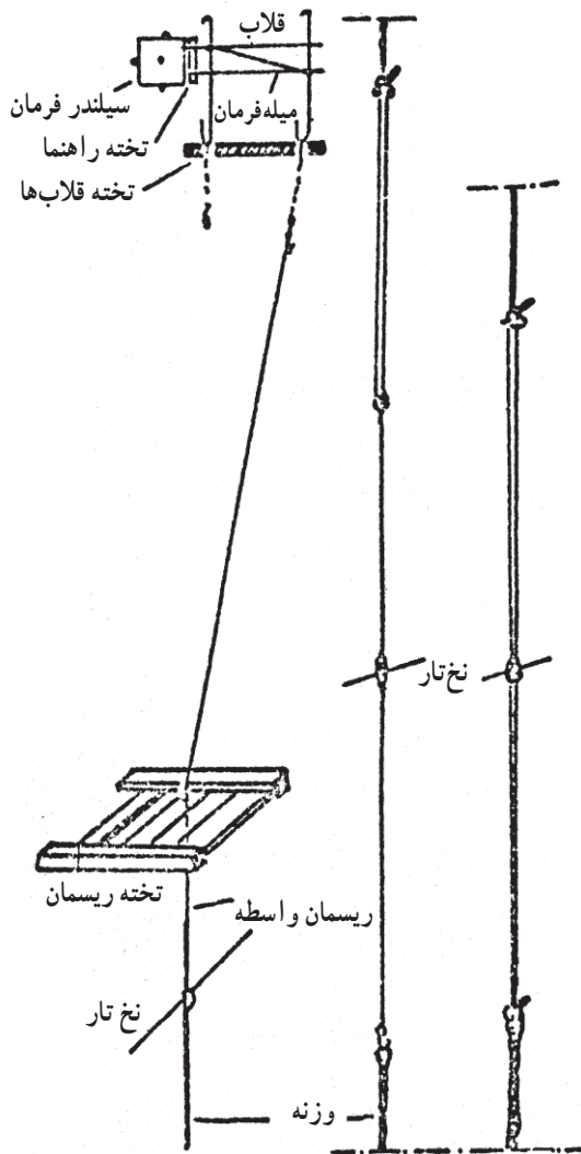
تصویر ۳۵- طرحی از مکانیزم دستگاه ژاکارد
