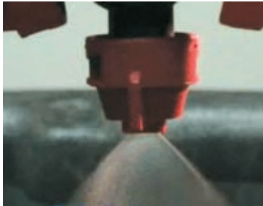
شکل ۲۴-۳- افشانک‌ها
