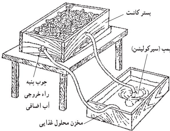
شکل ۷-۶- دستگاه هایدروپونیک بدون دستگاه تایمر
