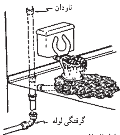
شکل ۱۱-۷- مشکلات احتمالی تخلیه آب باران در لوله فاضلاب
