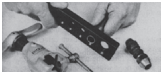
شکل ۲-۲۴- لاله کردن لوله‌ی مسی با لاله‌کن نوع پیچی
