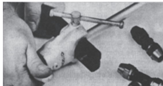
شکل ۲-۲۵- با چرخاندن پیچ (خروسک) لوله بین مرغک و بدنه قرار گرفته و لاله می‌شود.
