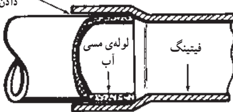
شکل ۲-۸- فاصله ی موینگی در اتصال لحیمی لوله کشی مسی
