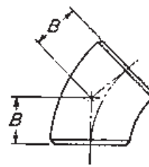
زانوی 45°
