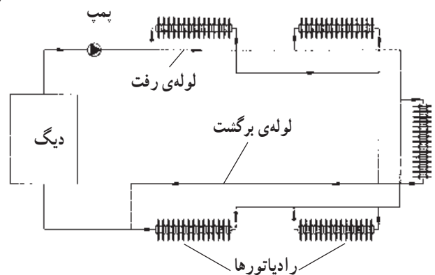
شکل ۶-۱- سیستم دو لوله‌ای با برگشت معکوس
