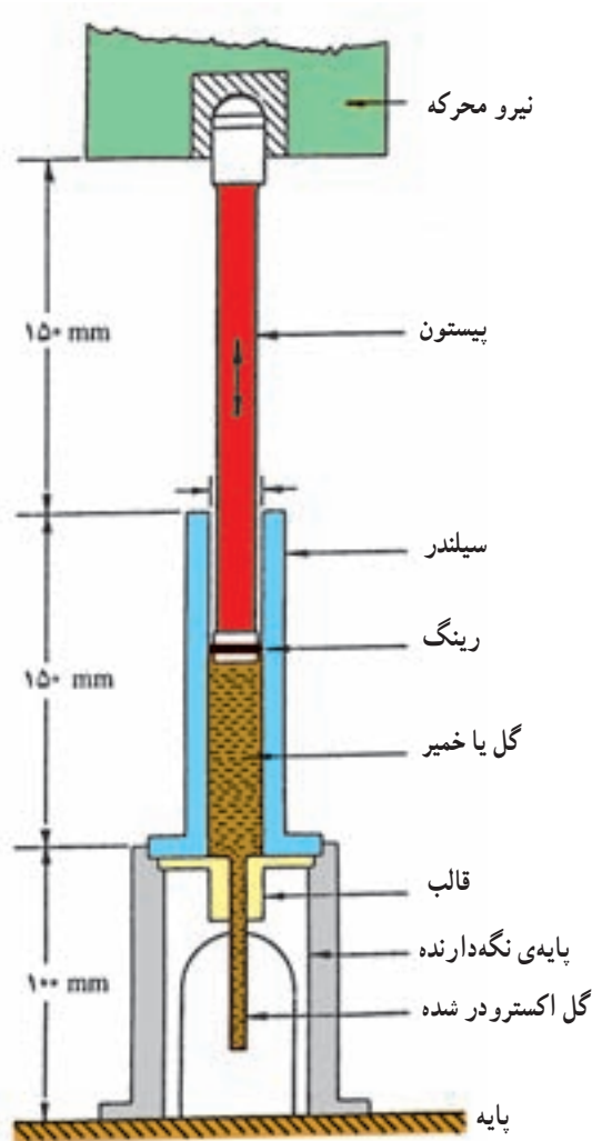
شکل ۱۷-۱- اکسترودر پیستونی
