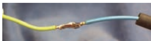
شکل ۱-۵۴- دو نمونه لحیم کاری قابل قبول
