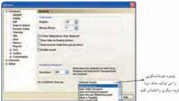
شکل ۵-۱ کادرمحاوره Options
