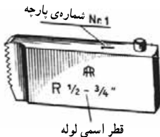
ب - مشخصات یک عدد پارچه‌ی حديدده، حديددهای چهار پارچه
