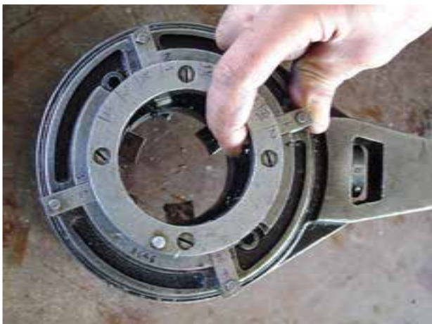
شکل ۴-۶۰- قرار دادن پارچه‌های مناسب در حدیده
