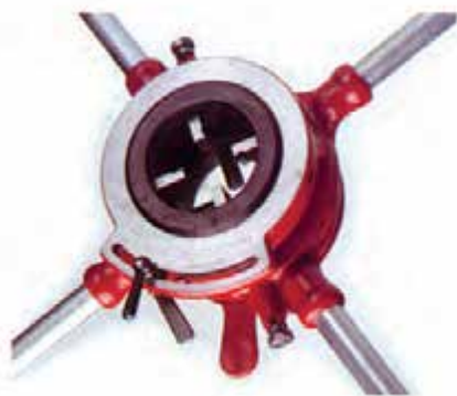
شکل ۴-۵۲- حديددهی چهار پارچه‌ی چهار دسته
