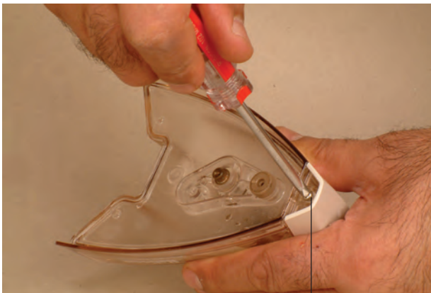
پیچ محکم کننده‌ی قاب پلاستیکی به بدنه‌ی مخزن
